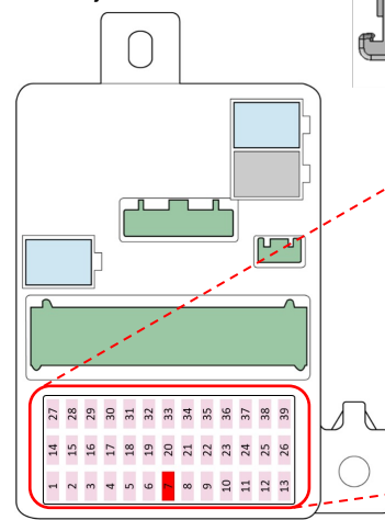
Sikringskasse under instrumentbrættet
