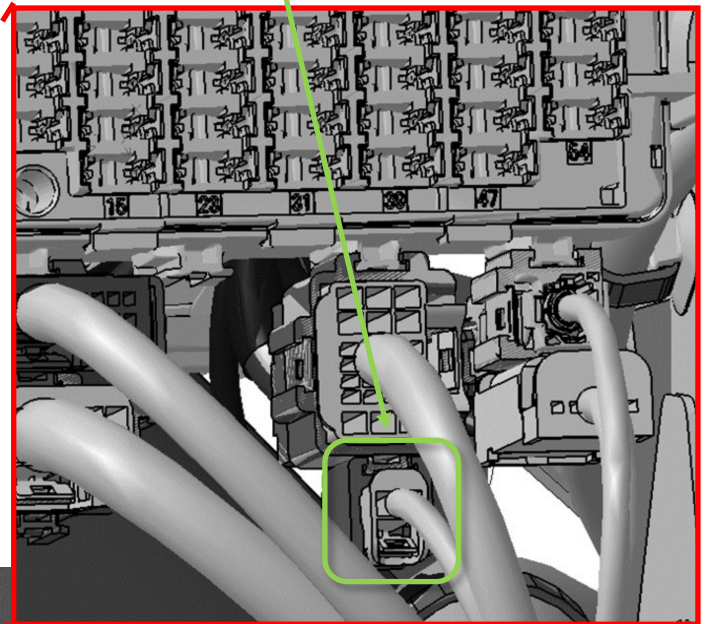
Connecteur fil-à-fil 2 broches
