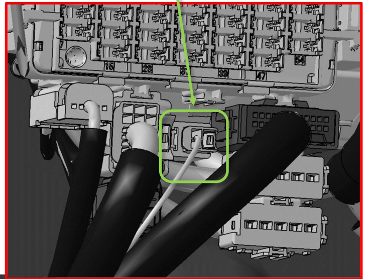
Conector de cable a cable de 2 pines
